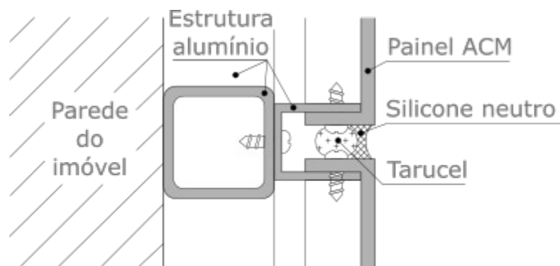
Detalhe da junta do ACM
